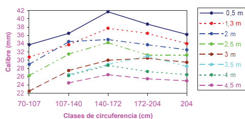
Figura 2 - Variación del calibre medido a diferentes alturas en función de la circunferencia normal (MONTERO y VALLEJO, 1990b)
