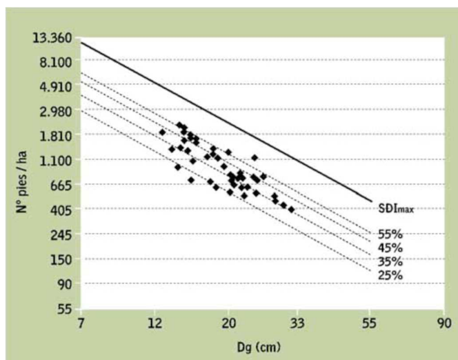
FIGURA 15: Recta de Reineke de máxima densidad (SDImax) para pino laricio y rectas del 25, 35, 45 y 55% de esta máxima densidad junto a los datos de las parcelas medidas en repoblaciones en Castilla y León.
