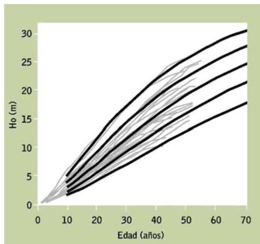
FIGURA 7: Datos de los análisis de tronco y curvas de calidad de estación.
