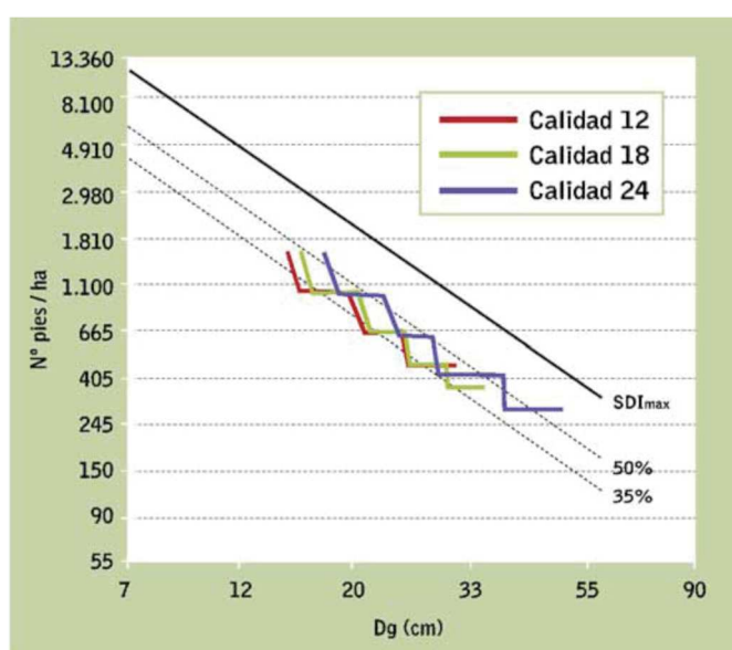
FIGURA 11: Propuesta selvícola para las calidades de estación 12, 18 y 24 junto con la recta de Reineke de máxima densidad (SDI max ) para pino silvestre y rectas del 35 y 50% de esta máxima densidad.
