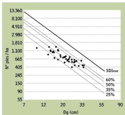
FIGURA 10: Recta de Reineke de máxima densidad (SDImax) para pino silvestre y rectas del 25, 35, 50 y 60% de esta máxima densidad junto a los datos de las parcelas medidas en repoblaciones en Castilla y León.
