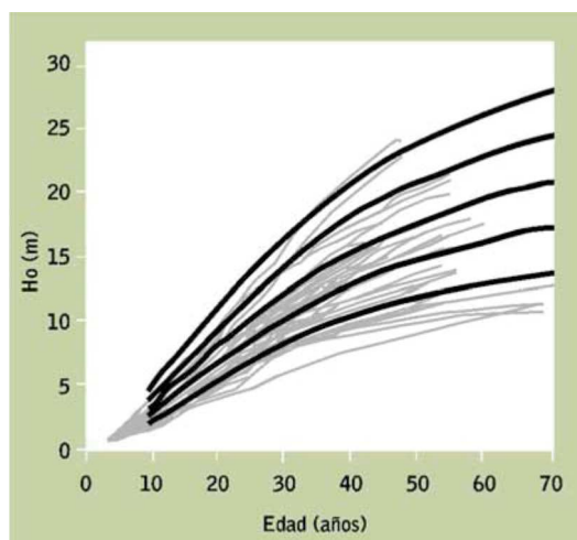
FIGURA 2: Datos de los análisis de tronco y curvas de calidad de estación.
