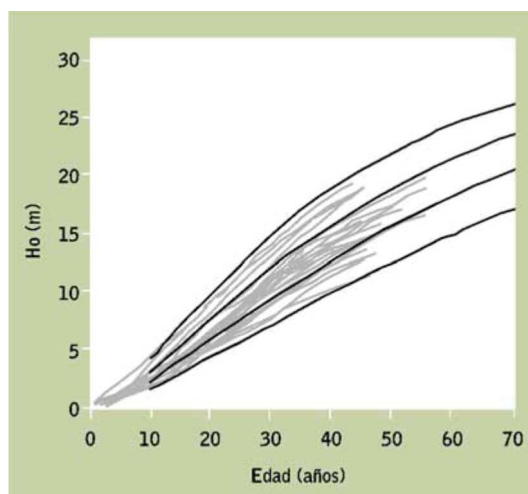
FIGURA 12 Datos de los análisis de tronco y curvas de calidad de estación.
